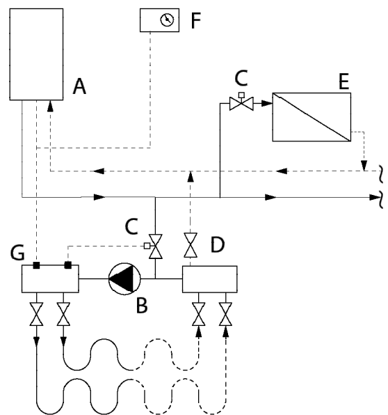
Aansluitschema vloerververming
