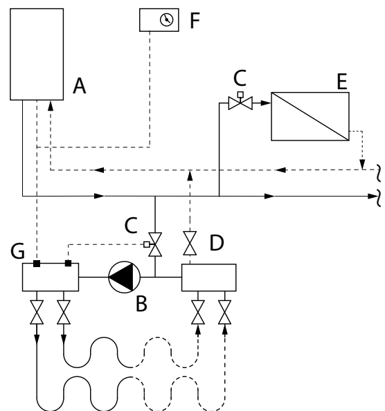
Aansluitschema vloerververming
