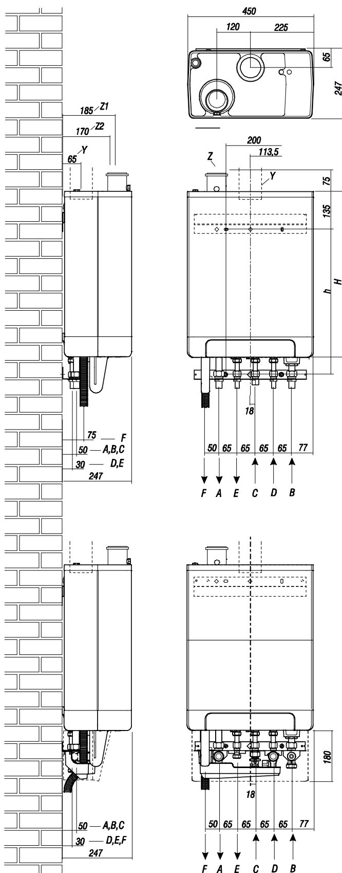
Toestel + montagebeugel
