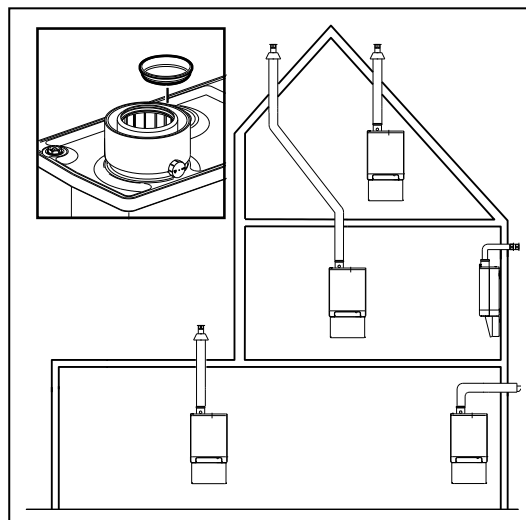
Concentrische aansluiting
