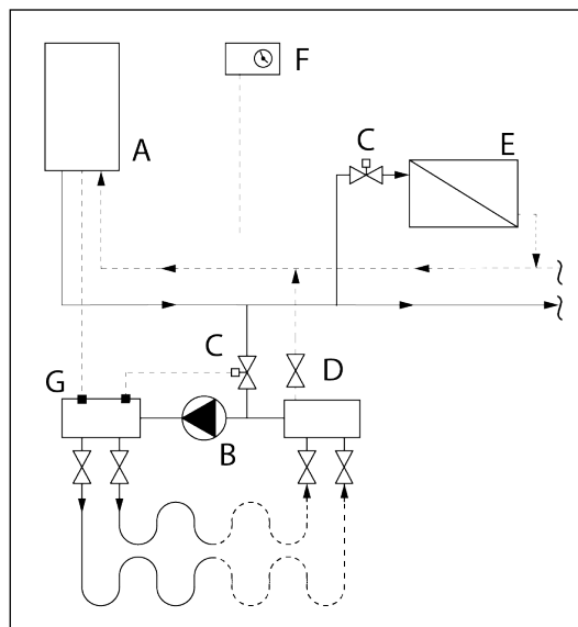
Aansluitschema vloerverwarming
