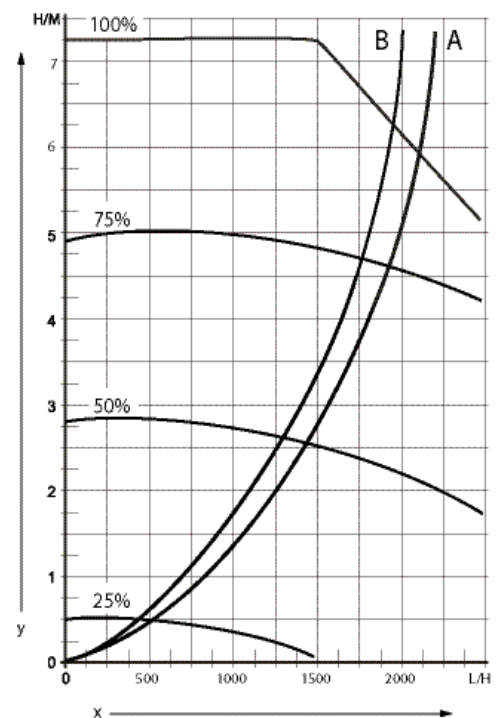
Pompkarakteristieken
